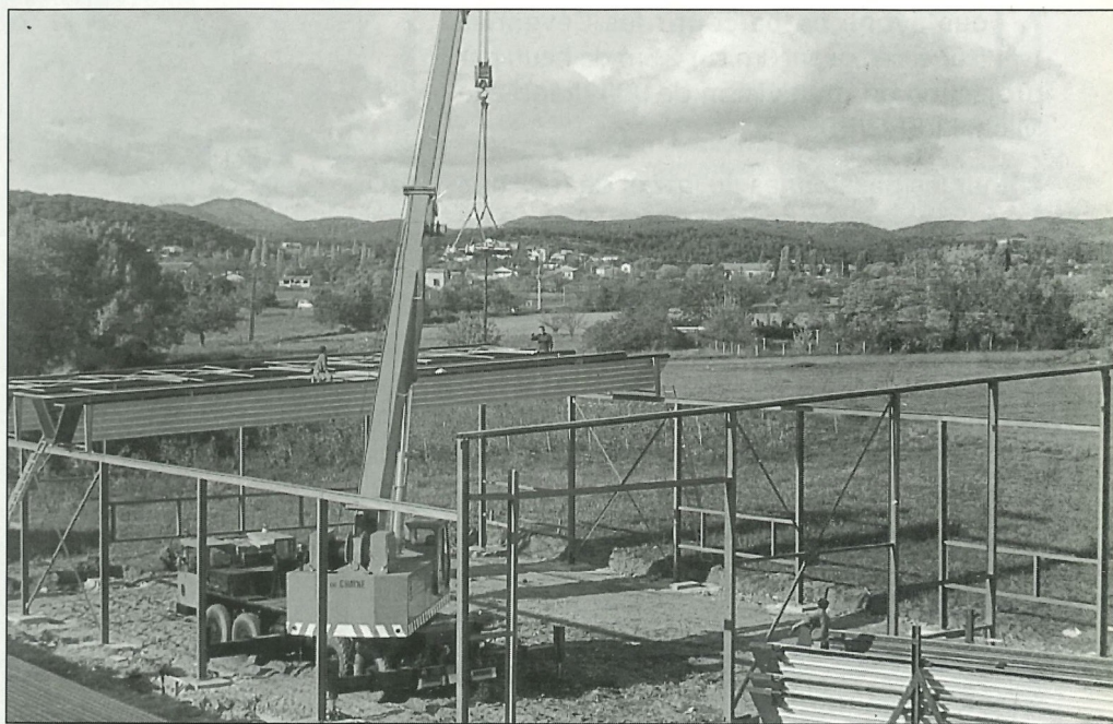
Première phase des travaux d'extension des ateliers au C.A.T. (terminés depuis). Photo : Midi-Libre
